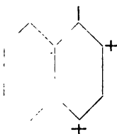
Disulfosäure für Naphtol- gelb. Bender. Ber. 22. 999.
